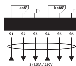
Przełączniki pomocnicze
