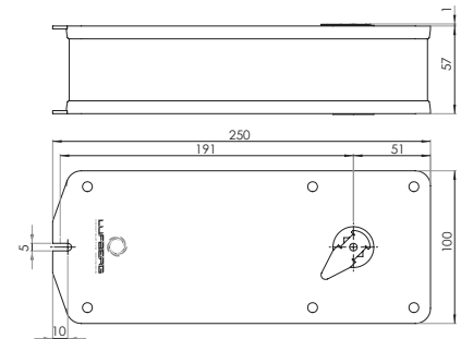
Włacznik termoelektryczny
