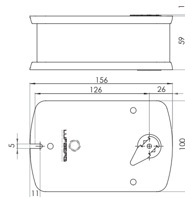
Włacznik termoelektryczny
