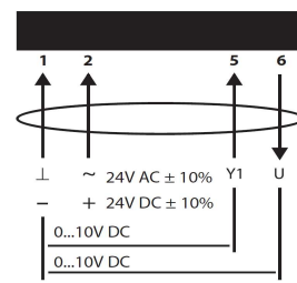
Электрическое подключение
